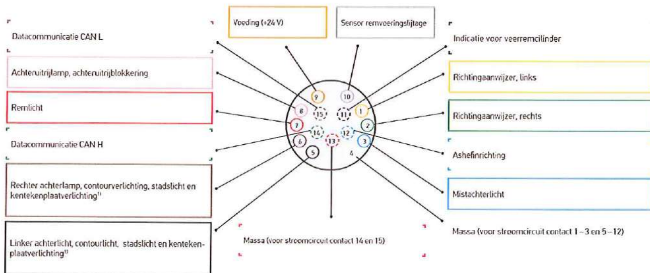
Contactbezetting voor stekkers conform ISO 12098, 24 V, 15-polig
